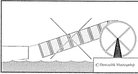
Şekil 3-a: Yanlış serme yöntemi
